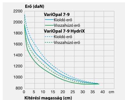
Erő-karakterisztika az orrbetétén
